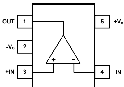
SOT-23-5
