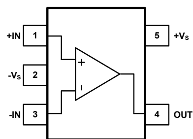
SOT-23-5
